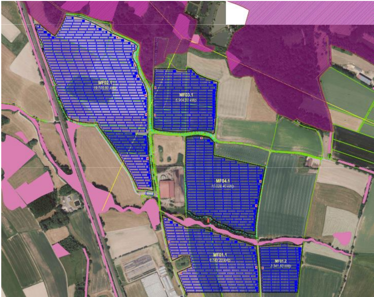
Abbildung 1: Anlagenlayout mit Modultischen
